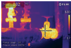
Zawór niezainstalowany
